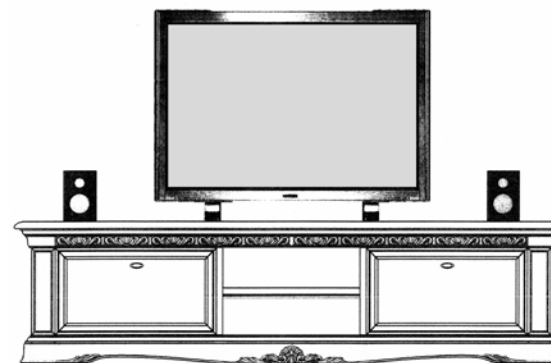
Art. 1752 Porta TV lungo TV cabinet, long Стенка для телевизора, длинная 213 x 59 x 57 cm 83,92 x 23,25 x 22,46 inch nr. colli / nr. of items / количество грузовых мест: 1 m³: 0,87 peso netto / net weight / вес нетто: 83 kg peso lordo / gross weight / вес брутто: 90 kg
